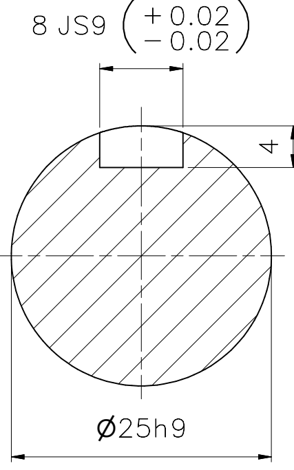
C-C ( 2 : 1 )
