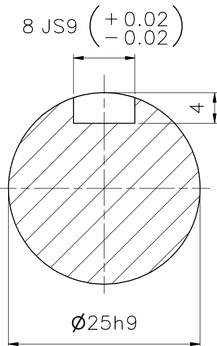
B-B ( 2 : 1 )
